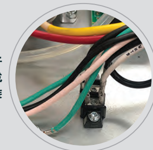
高压接线端子 用于有线或 硬连接安装
