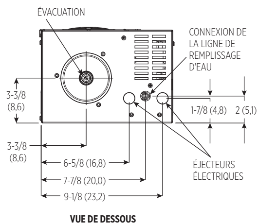
FIGURE 3 – DIMENSIONS DU BLOC VENTILATEUR (POUCES [CM])
