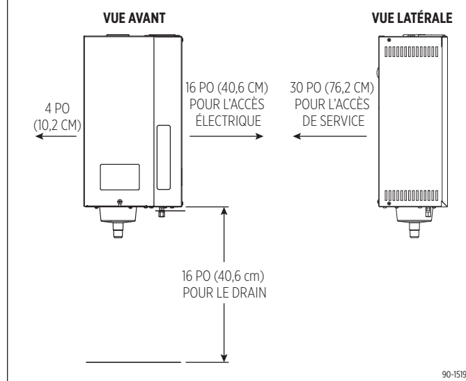
FIGURE 11 – DÉGAGEMENTS
