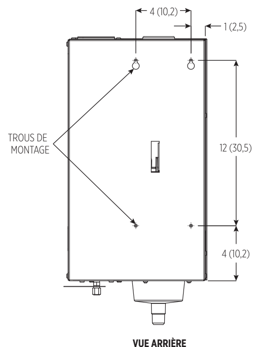
FIGURE 3 – DIMENSIONS DU BLOC VENTILATEUR (POUCES [CM])
