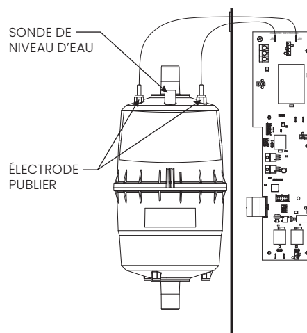
FIGURE 17 – EMPLACEMENT DE L'ÉLECTRODE
