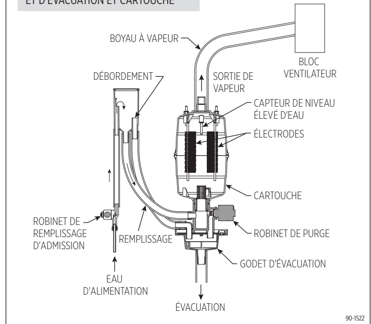
FIGURE 1 – SYSTÈME DE REMPLISSAGE ET D'ÉVACUATION ET CARTOUCHE
