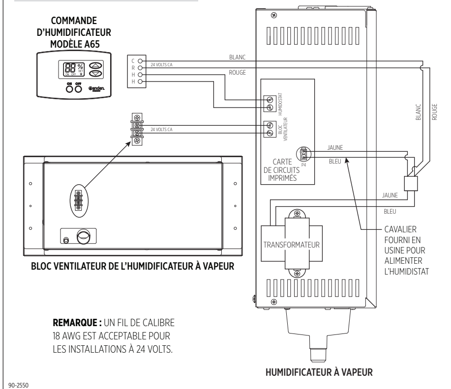
FIGURE 15 – CÂBLAGE DU MODÈLE A65
