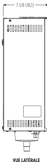
FIGURE 3 – DIMENSIONS DU BLOC VENTILATEUR (POUCES [CM])
