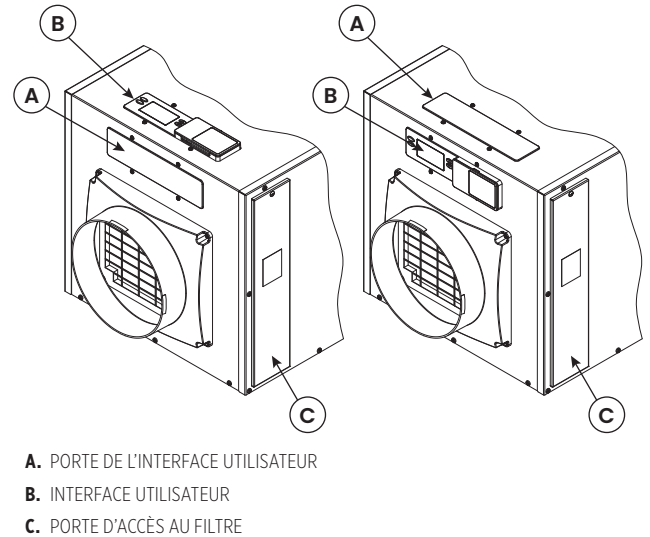
FIGURE 3 : EMPLACEMENT DE L'INTERFACE UTILISATEUR
