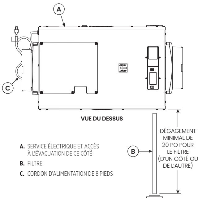
FIGURE 5 : DÉGAGEMENT POUR L'ACCÈS AU FILTRE
