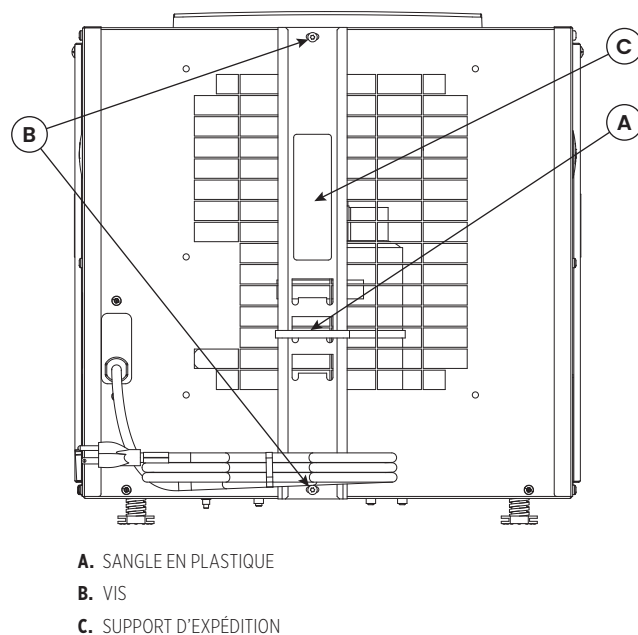
FIGURE 1 : PRÉPARATION DE L'APPAREIL POUR L'INSTALLATION
