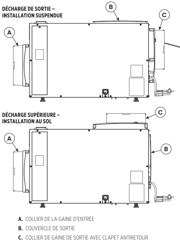
FIGURE 2 : INSTALLATIONS ENTièrement GAINÉES
