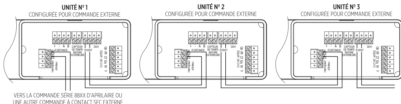
FIGURE 14 : CÂBLAGE EN GUIRLANDE AVEC COMMANDE EXTERNE ALTERNATIVE
