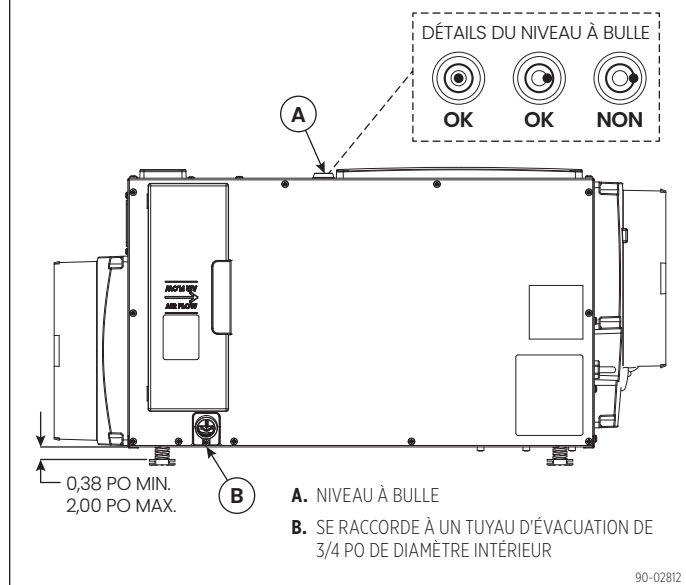
FIGURE 7 : MISE À NIVEAU DE L'APPAREIL
