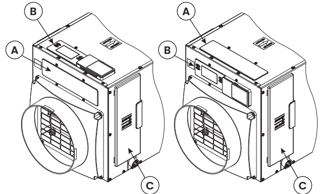
FIGURE 3 : EMPLACEMENT DE L'INTERFACE UTILISATEUR
