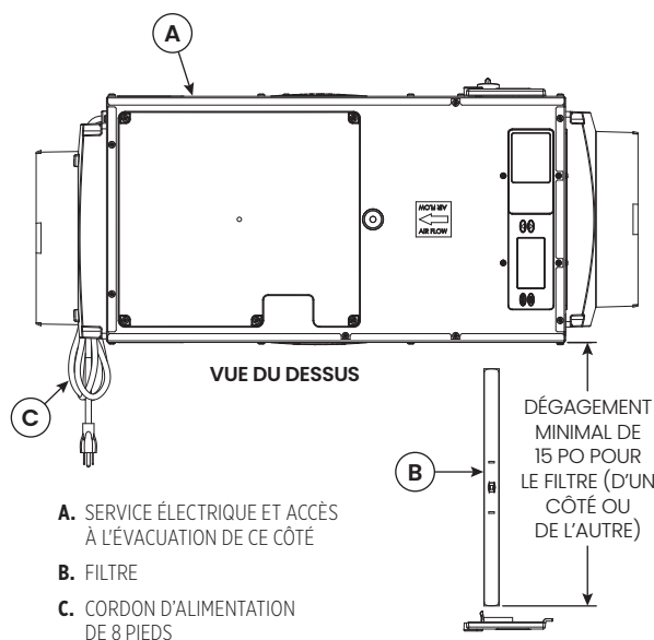
FIGURE 5 : DÉGAGEMENT POUR L'ACCÈS AU FILTRE
