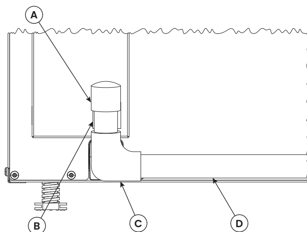
FIGURE 6 : ACCÈS À L'ÉVACUATION À BOUCHON POUR LE NETTOYAGE
