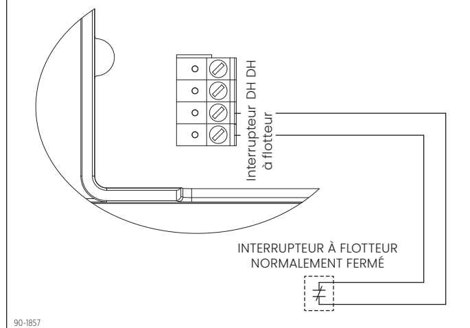
FIGURE 8 : CÂBLAGE DE L'INTERRUPTEUR À FLOTTEUR
